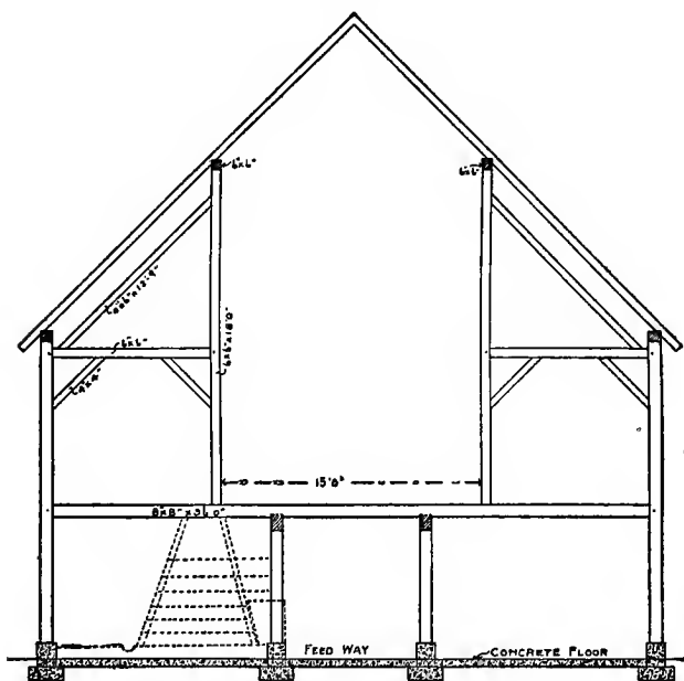
Fig. 127. Center Bent of Hay Barn.
