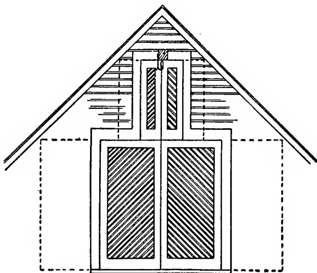
Fig. 142. Double Hay-Mow Doors.
